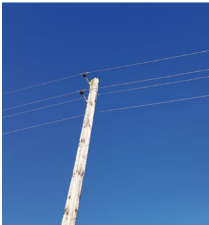
Niederspannung: Blanke Freileitung
